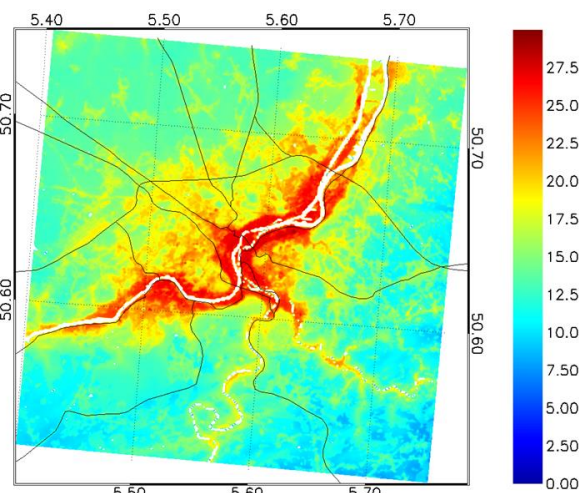
Prédiction du nombre de jours de canicule par été pour la période 2081-2100 selon UrbClim
