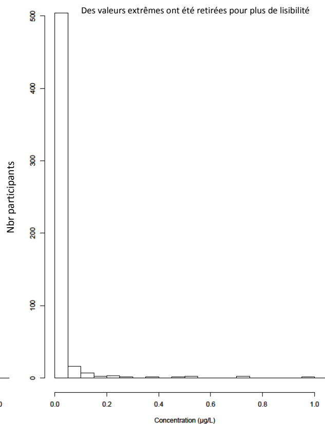
BPZ
