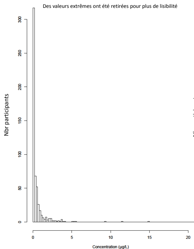
BPS
