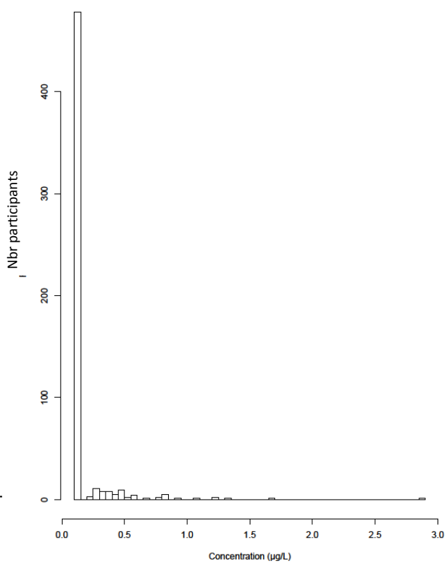
Hg
