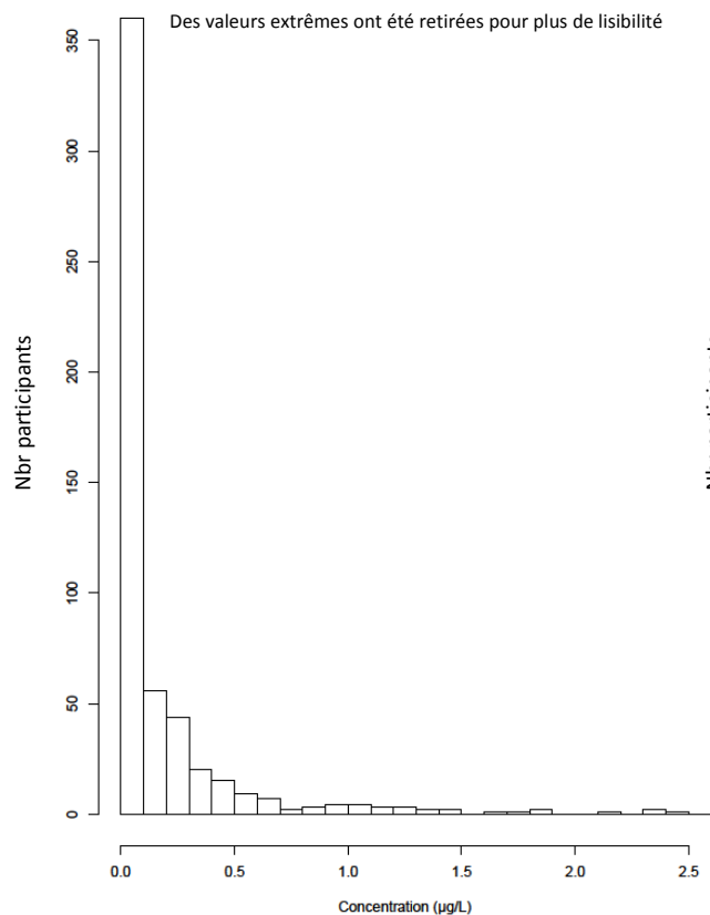
BPS
