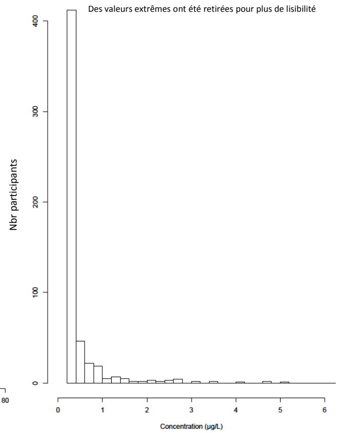
DMTP
