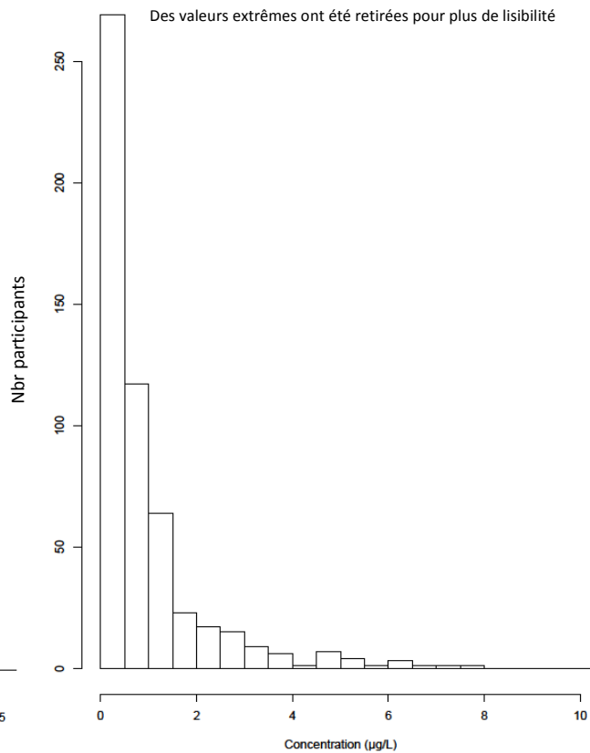
BPZ
