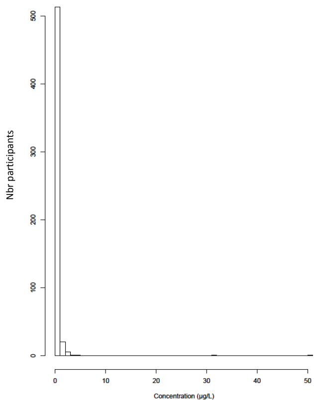
c-DCCA
