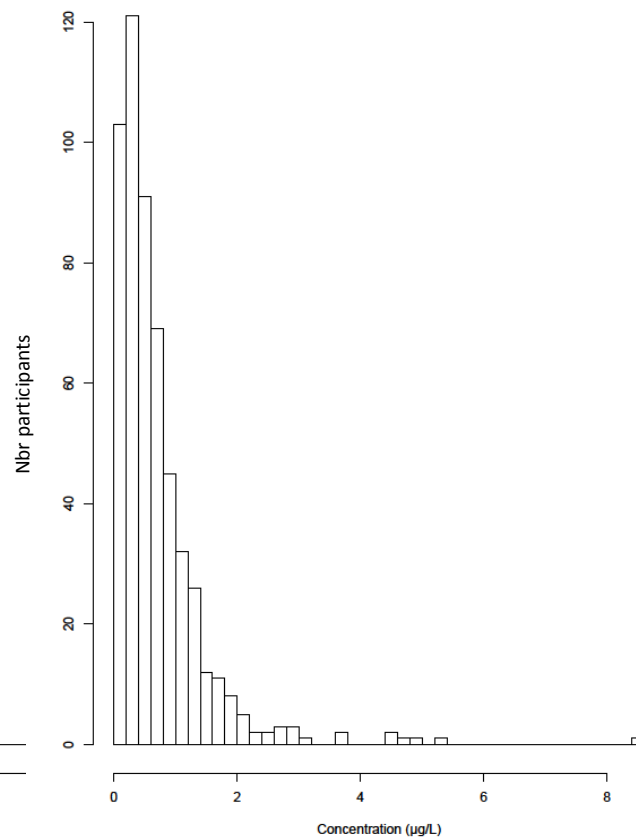
t-DCCA
